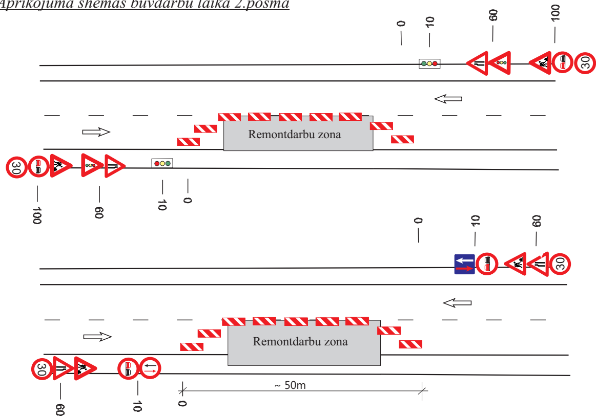
Aprīkojuma shēmas būvdarbu laikā 2.posmā
